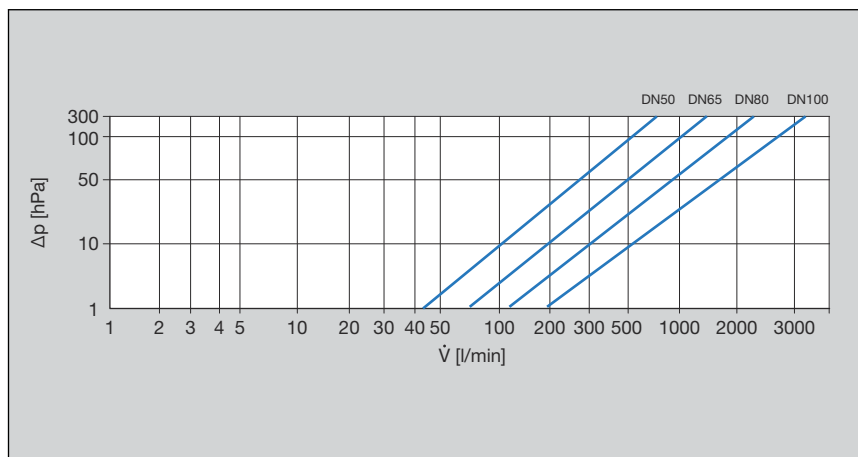
Fig. 1: Diagramme de performances perte de charge KRV vannes à siège incliné XL raccord par bride
