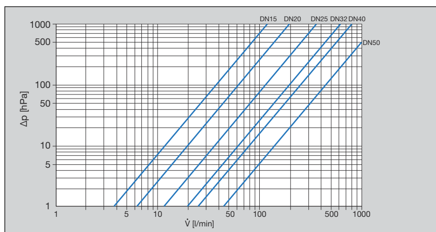
Fig. 1: Diagramme de performances vannes à siège incliné raccord à sertir/raccordement fileté
