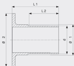
Seapress kaulus - CuNiFe malli 0359.3
