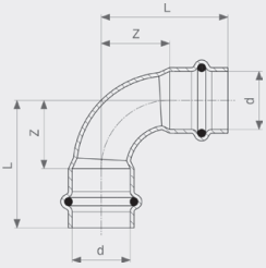
Seapress käyrä 90° - CuNiFe malli 0316
