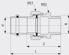
Seapress yhdistäjä - CuNiFe malli 0365
