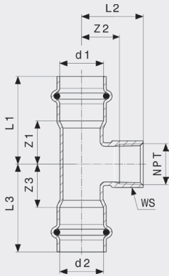
Seapress T-yhde - CuNiFe malli 0317.5
