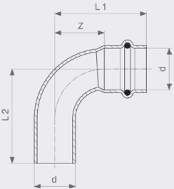
Seapress käyrä 90° - CuNiFe malli 0316.1
