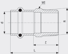
Seapress nippa - CuNiFe malli 0311
