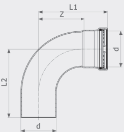
Seapress XL käyrä 90° - CuNiFe malli 0316.1XL
