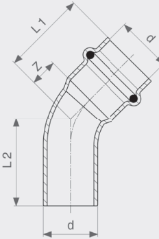
Seapress käyrä 45° - CuNiFe malli 0326.1
