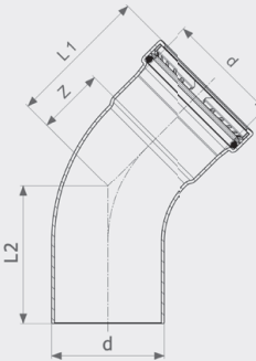
Seapress XL käyrä 45° - CuNiFe malli 0326.1XL
