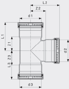
Seapress T-yhde - CuNiFe malli 0318
