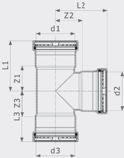
Seapress XL T-yhde - CuNiFe malli 0318XL
