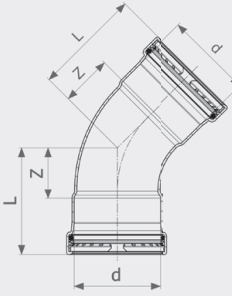
Seapress XL käyrä 45° - CuNiFe malli 0326XL
