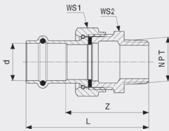
Seapress yhdistäjä - CuNiFe malli 0365.5
