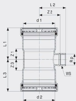
Seapress T-yhde - CuNiFe malli 0317.2
