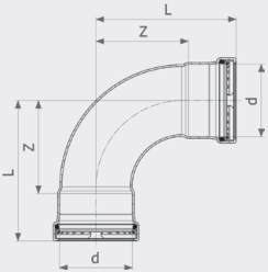
Seapress XL käyrä 90° - CuNiFe malli 0316XL
