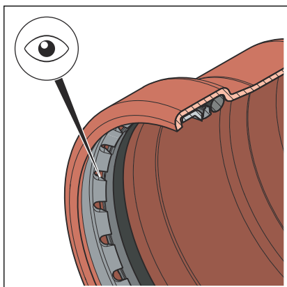
Fig. 6: Anillo cortante
