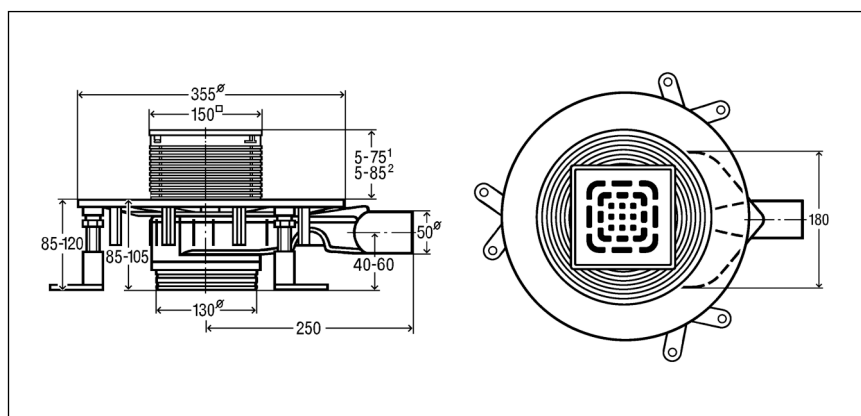
Fig. 7: Dibujo acotado del modelo 4914.21
