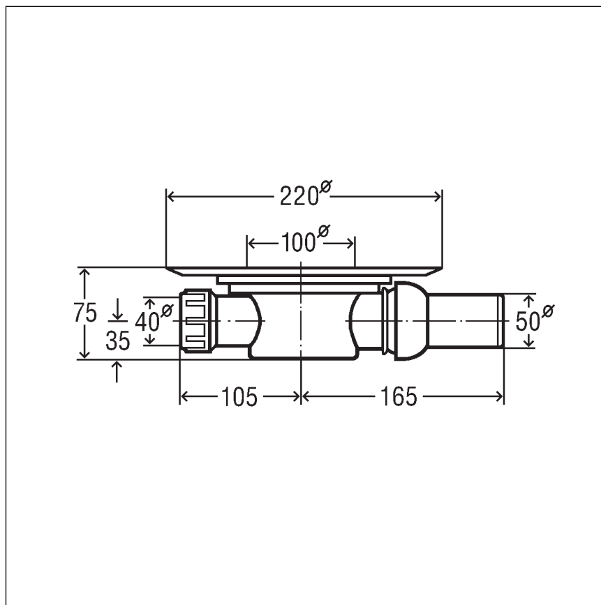
Fig. 7: Dibujo acotado del modelo 4935.6
