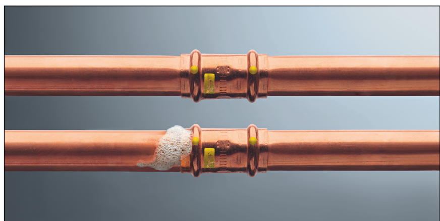
Fig. 2: SC-Contur
