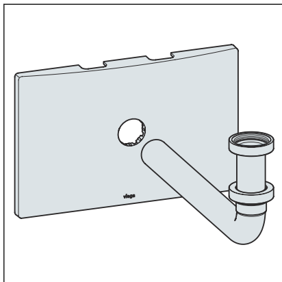
Abdeckplatte für UP-Anschlussbox Modell 8314.5
