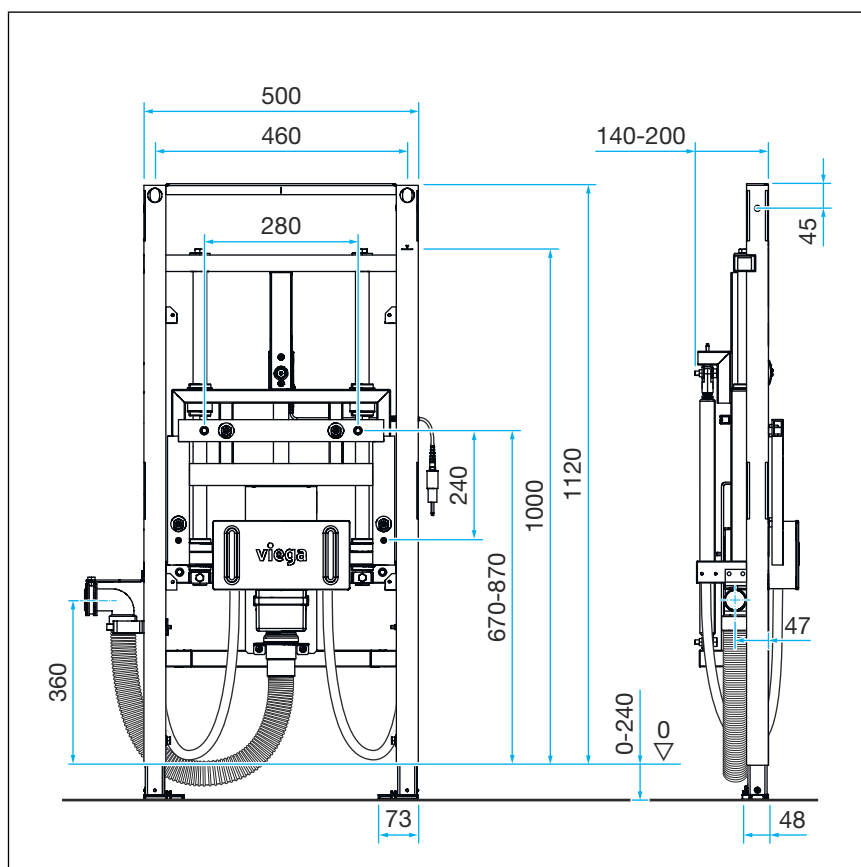
Abb. 3: Abmessungen
