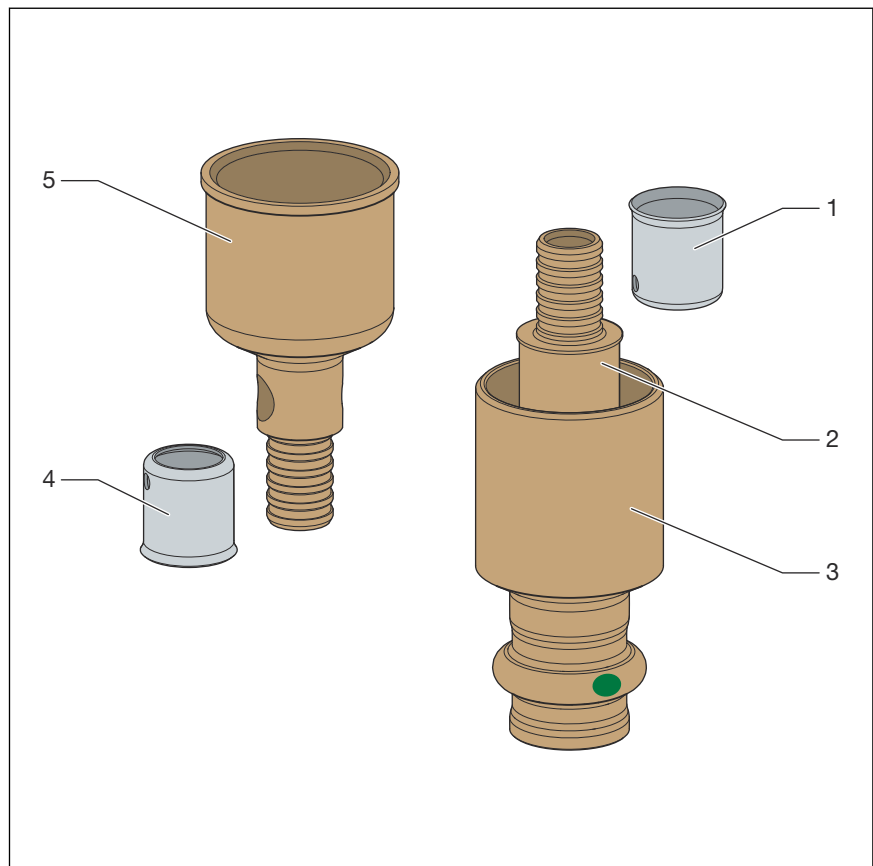
Abb. 1: Anschlussset, Modell 2276.1
