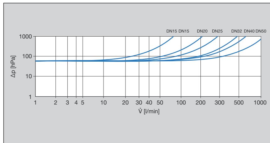
Abb. 3: Leistungsdiagramm Druckverlust RV Press-/Gewindeanschluss
