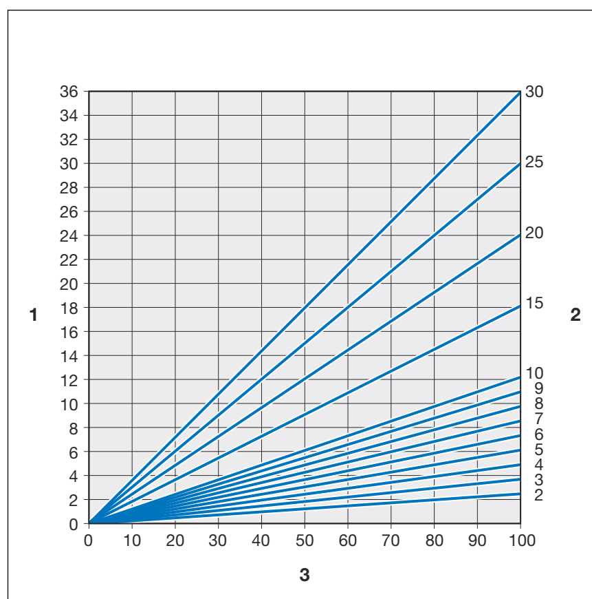
Abb. 3: Längenausdehnung Stahlrohre
