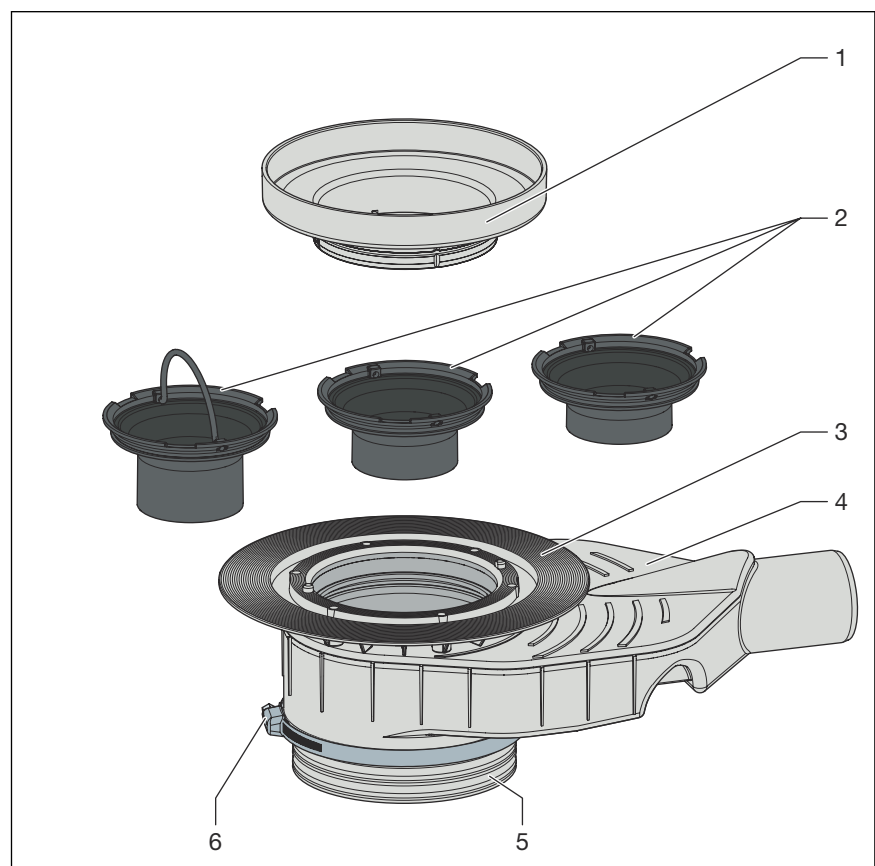
Abb. 1: Lieferumfang Modell 4927.3
