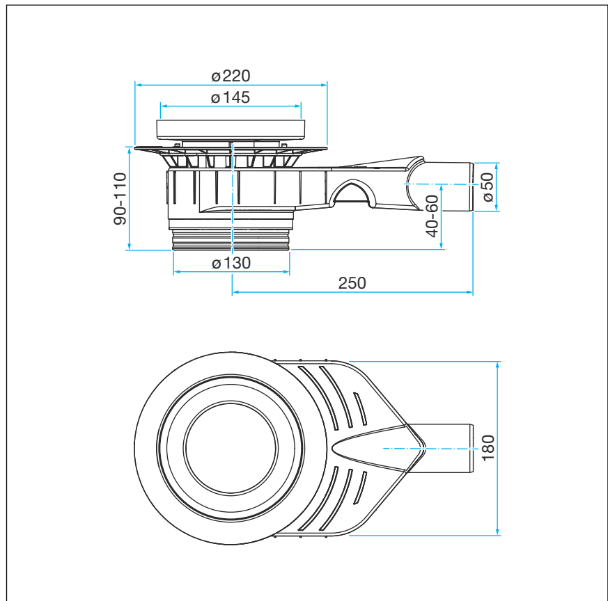
Abb. 8: Maßzeichnung Modell 4927.3
