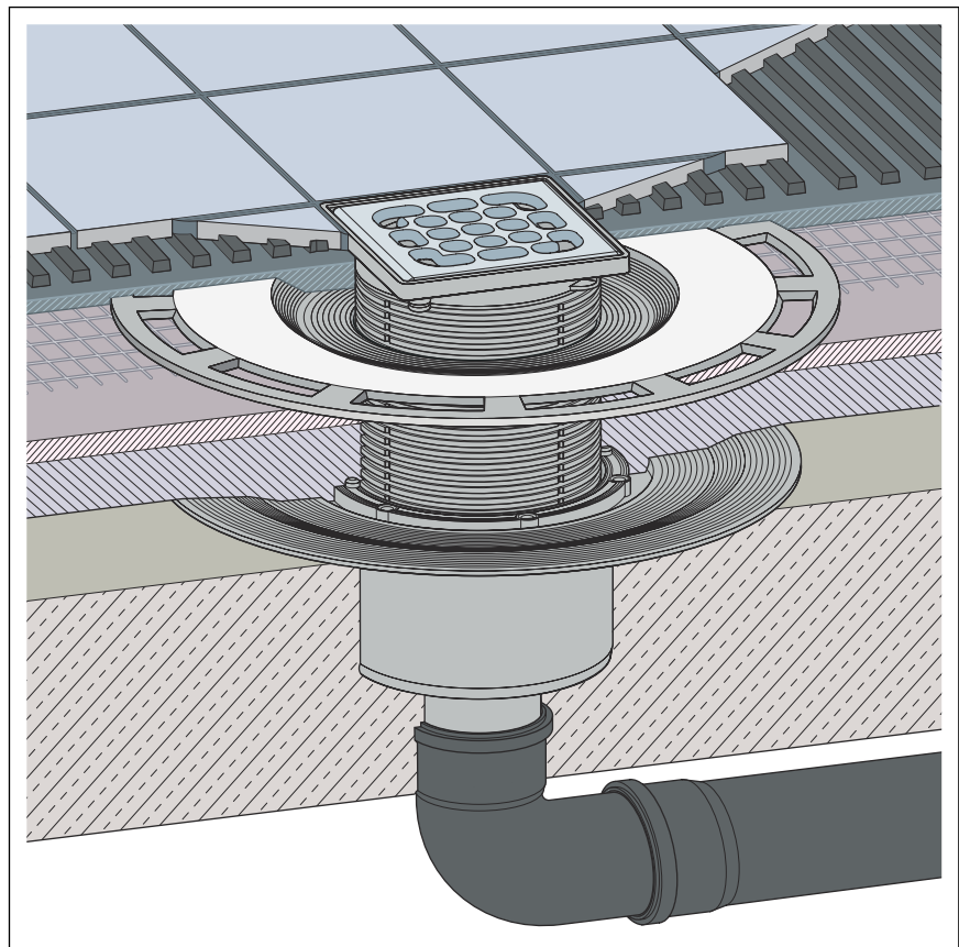
Abb. 5: Schema einer Verbundabdichtung mit Aufstockelement
