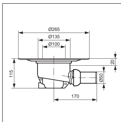
Abb. 7: Maßzeichnung Modell 4921.3
