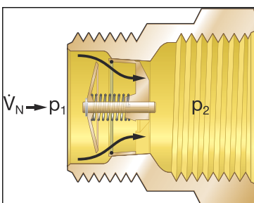
Abb. 3: Normalbetrieb
