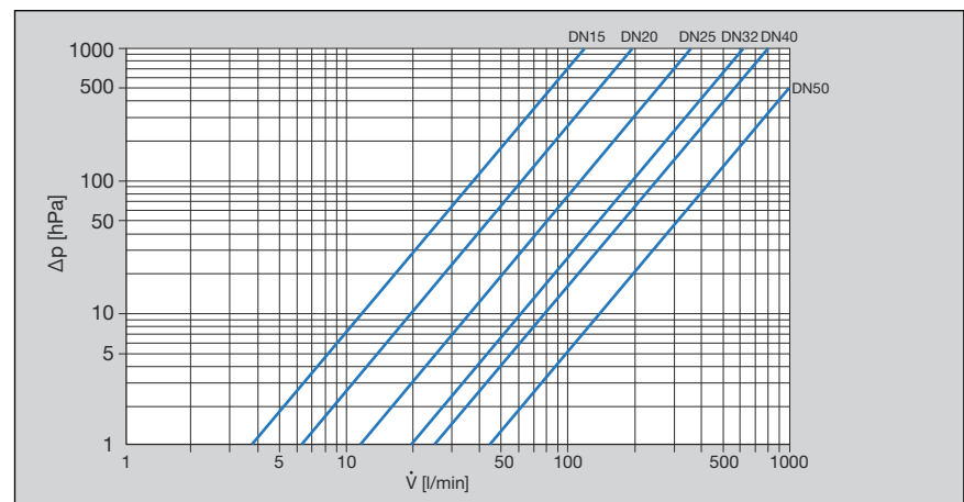
Abb. 1: Leistungsdiagramm Schrägsitzventile Press-/Gewindeanschluss
