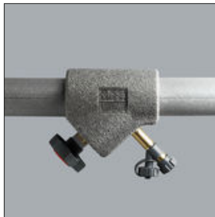
Abb. 4: Easytop-Dämmschale mit Verlängerung und Entleerungsventil
