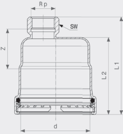
Sanpress Inox XL LF-Kappe - Stahl nichtrostend Modell 2356XLLF
