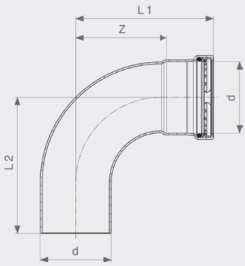
Sanpress Inox XL LF-Bogen 90° - Stahl nichtrostend Modell 2316.1XLLF
