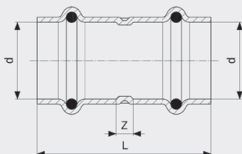
Sanpress Inox LF-Muffe - Stahl nichtrostend Modell 2315LF
