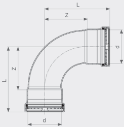
Sanpress Inox XL LF-Bogen 90° - Stahl nichtrostend Modell 2316XLLF
