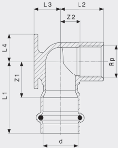
Sanpress Inox LF-Wandscheibe - Stahl nichtrostend Modell 2325.5LF
