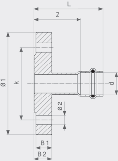
Sanpress Inox LF-Flanschübergang - Stahl nichtrostend Modell 2359LF
