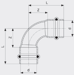
Sanpress Inox LF-Bogen 90° - Stahl nichtrostend Modell 2316LF
