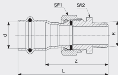
Sanpress Inox LF-Übergangverschraubung - Stahl nichtrostend Modell 2365LF
