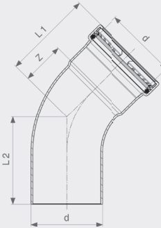
Sanpress Inox XL LF-Bogen 45° - Stahl nichtrostend Modell 2326.1XLLF
