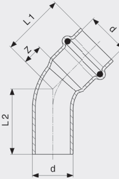
Sanpress Inox LF-Bogen 45° - Stahl nichtrostend Modell 2326.1LF
