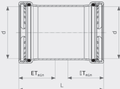
Sanpress Inox XL LF-Schiebemuffe - Stahl nichtrostend Modell 2315.5XLLF
