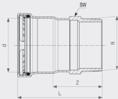
Sanpress Inox XL LF-Übergangsstück - Stahl nichtrostend Modell 2311XLLF
