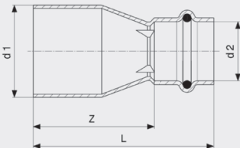
Sanpress Inox LF-Reduzierstück - Stahl nichtrostend Modell 2315.1LF
