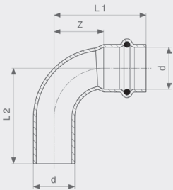
Sanpress Inox LF-Bogen 90° - Stahl nichtrostend Modell 2316.1LF
