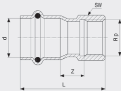
Sanpress Inox LF-Übergangsstück - Stahl nichtrostend Modell 2312LF
