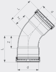
Sanpress Inox XL LF-Bogen 45° - Stahl nichtrostend Modell 2326XLLF
