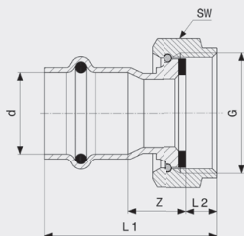
Sanpress Inox LF-Anschlussverschraubung - Stahl nichtrostend Modell 2363LF
