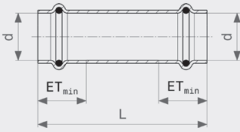
Sanpress Inox LF-Schiebemuffe - Stahl nichtrostend Modell 2315.5LF
