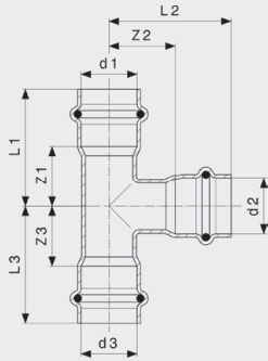
Sanpress Inox LF-T-Stück - Stahl nichtrostend Modell 2318LF
