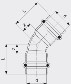
Sanpress Inox LF-Bogen 45° - Stahl nichtrostend Modell 2326LF
