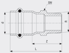
Sanpress Inox LF-Übergangsstück - Stahl nichtrostend Modell 2311LF
