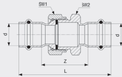
Sanpress Inox LF-Verschraubung - Stahl nichtrostend Modell 2360LF
