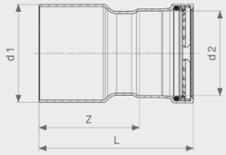
Sanpress Inox XL LF-Reduzierstück - Stahl nichtrostend Modell 2315.1XLLF
