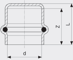
Sanpress Inox LF-Kappe - Stahl nichtrostend Modell 2356LF
