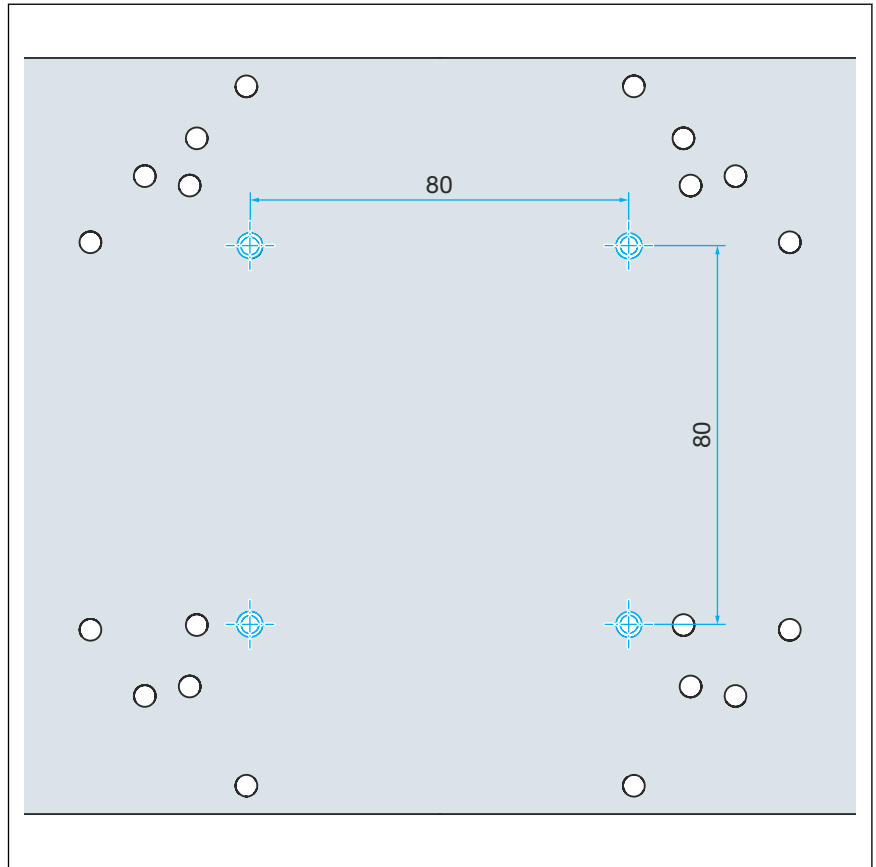
Abb. 4: Hansa HANSAVAROX
