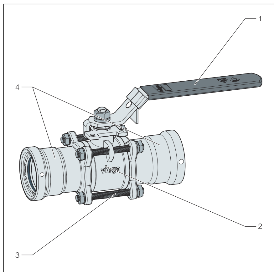
Abb. 2: dreiteiliger Kugelhahn
