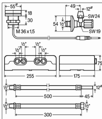
Abb. 6: Abmessungen
