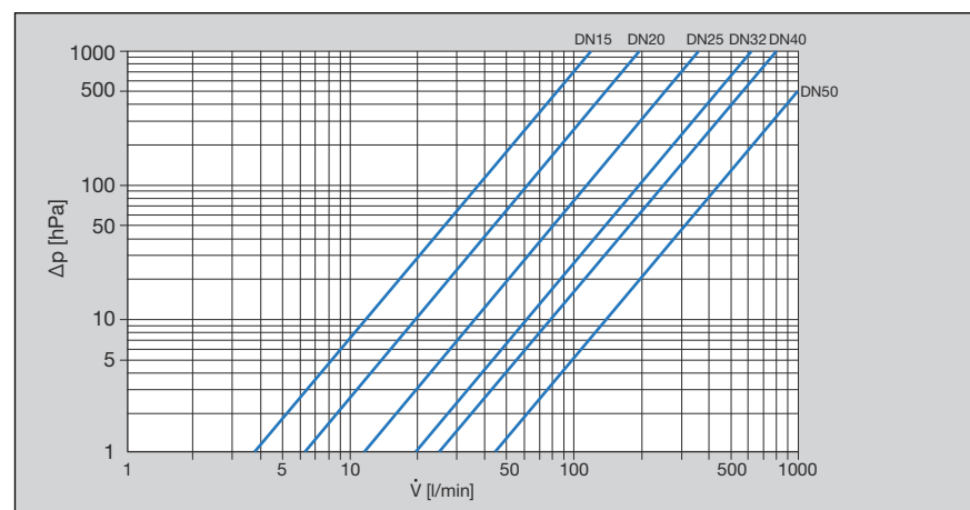
Fig. 1: Effektdiagram skrånedeventiler pres-/gevindtilslutning
