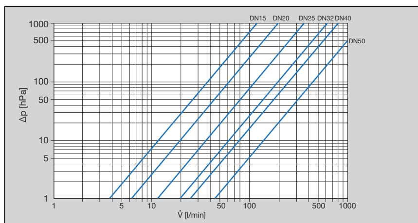
Fig. 1: Effektdiagram skrånedeventiler pres-/gevindtilslutning
