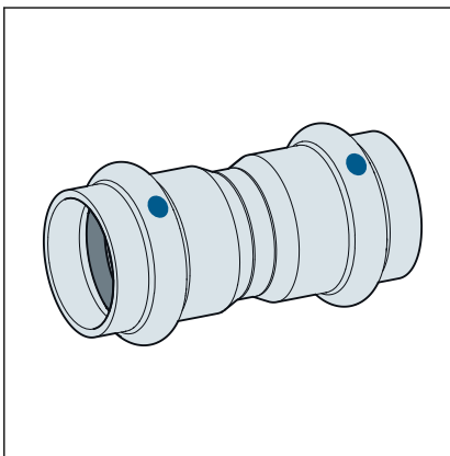
Fig. 5: Mærkning på presfittingsen
