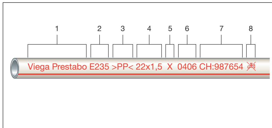
Fig. 7: Rør med PP-kappe
