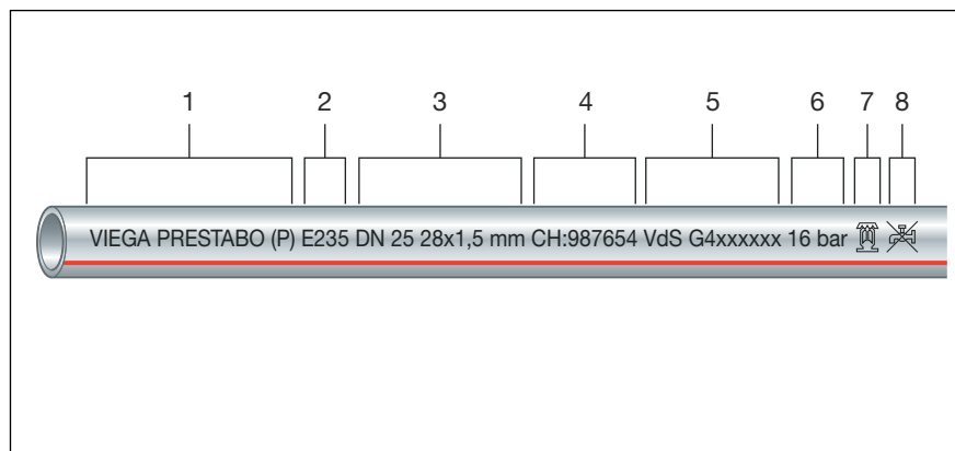
Fig. 8: Rør ind- og udvendigt sendzimirgalvaniseret
