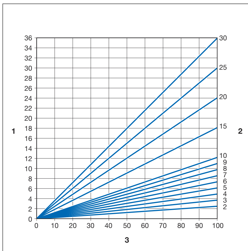
Fig. 3: Længdeudvidelse stålrør
