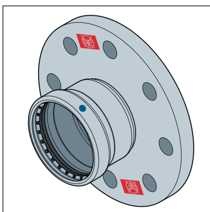
Fig. 11: Fast flange 1159XLLF
