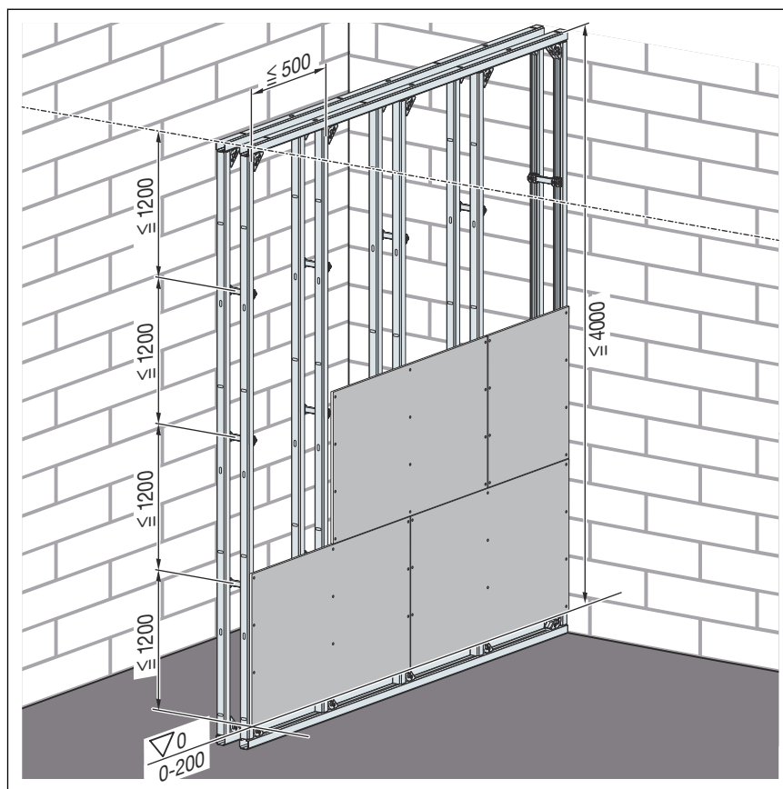
Rámové konstrukce Steptec obložte jednou vrstvou.
