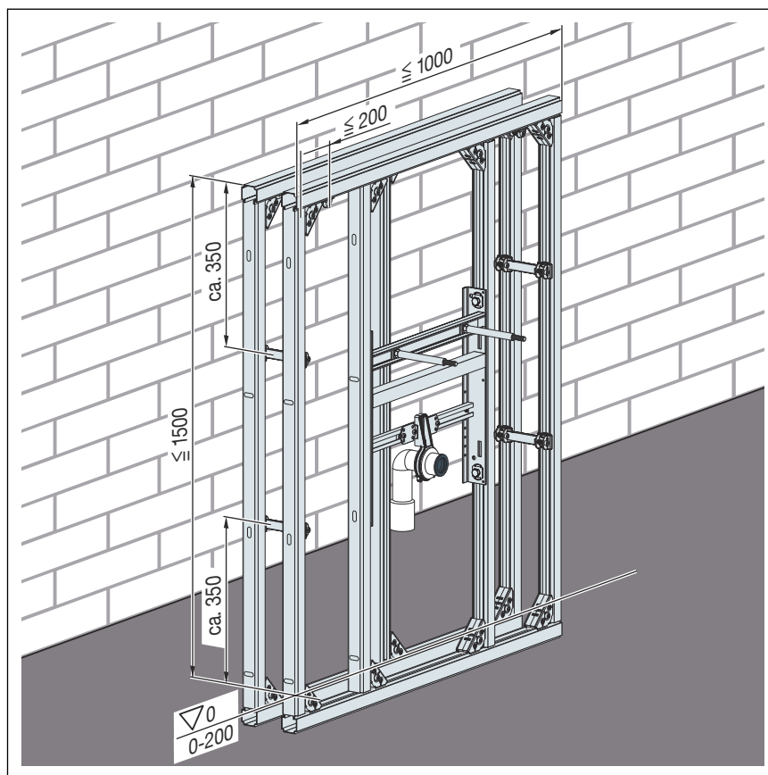
Volně stojící dělicí stěna
