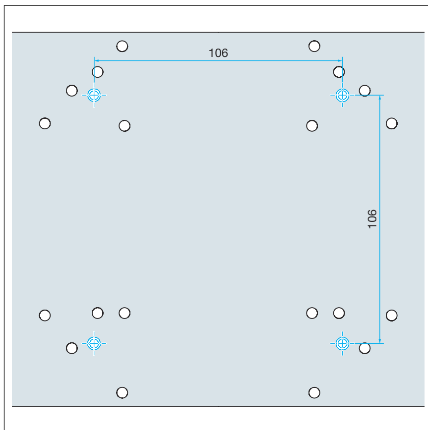
Obr. 5: Hansgrohe „I-Box“
