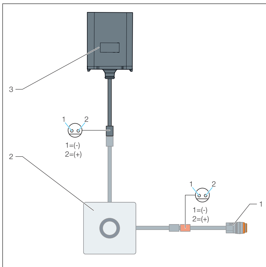
Obr. 1: schéma připojení, zásobník na baterie, pisoárová ovládací deska Prevista
