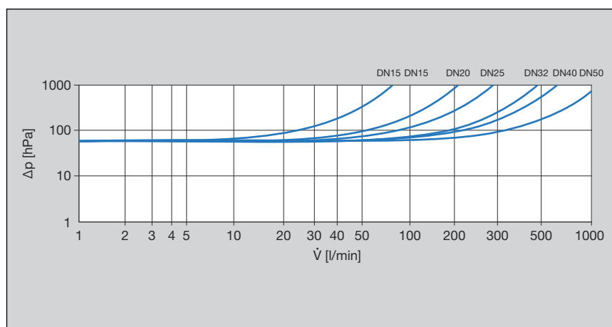
Obr. 3: výkonový diagram tlakové ztráty zamezovače zpětného toku lisovací/závitový přípoj
