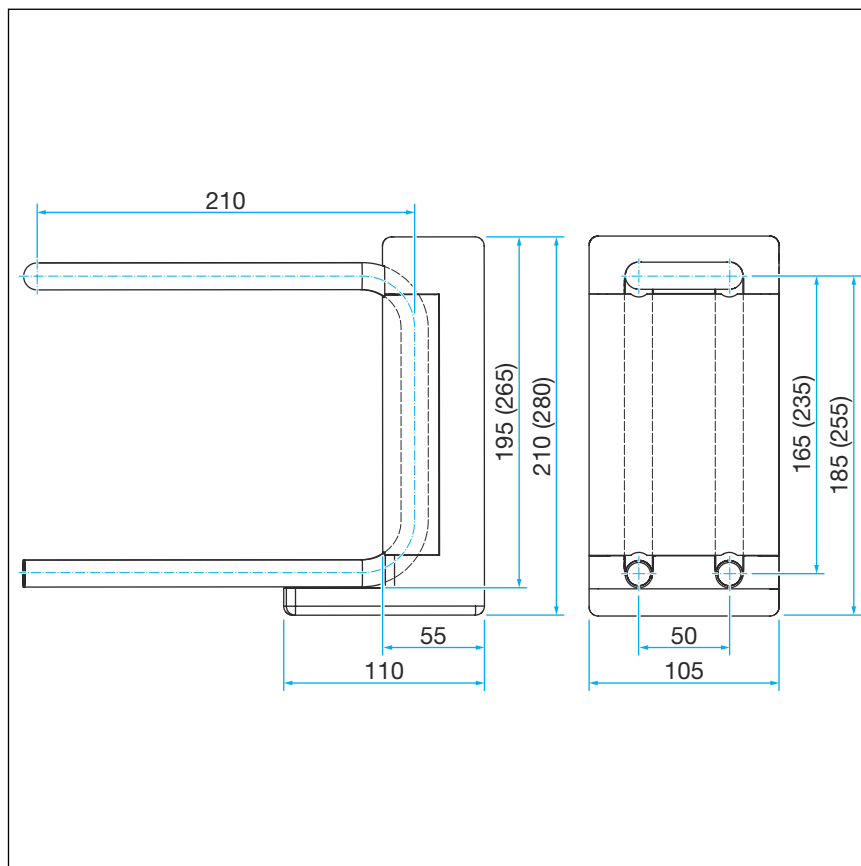
Obr. 1: montážní rozměry
