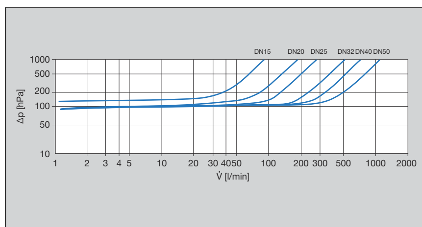
Obr. 3: výkonový diagram tlakové ztráty KRV lisovací/závitový přípoj
