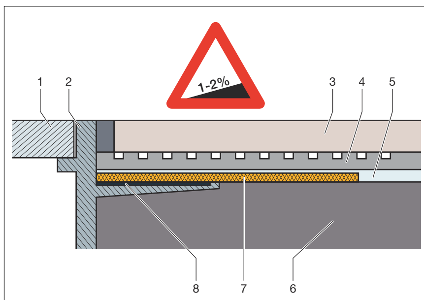
Obr. 11: Schéma konstrukce spojené izolace – sklon potěru min. 1–2 %
