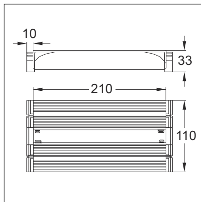
Obr. 4: rozměry spojovacího kusu
