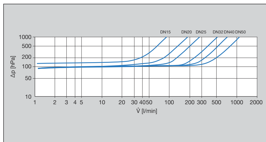
Obr. 1: výkonový diagram tlakové ztráty KRV lisovací/závitový přípoj
