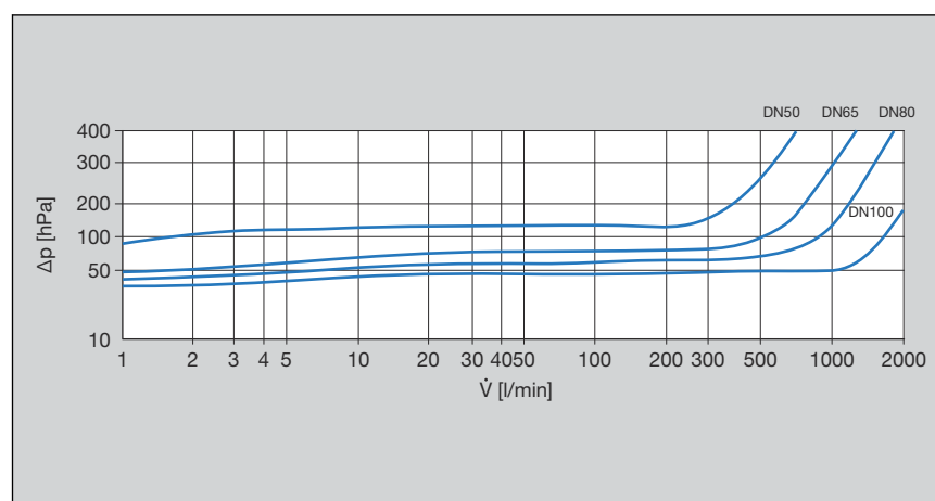
Obr. 1: výkonový diagram tlakové ztráty zamezovače zpětného toku přírubový přípoj
