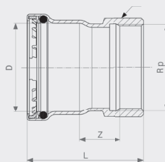
Megapress S XL-přechodový kus - nelegovaná ocel, povrchová úprava zinek-nikl model 4212XL
