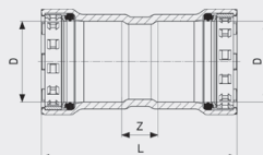
Megapress S-objímka - nelegovaná ocel, povrchová úprava zinek-nikl model 4315
