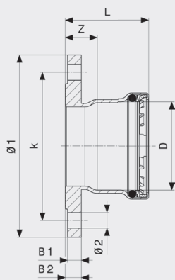
Megapress S XL-přírubový přechod - nelegovaná ocel, povrchová úprava zinek-nikl model 4259.6XL
